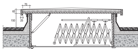
type 2470 gesloten
