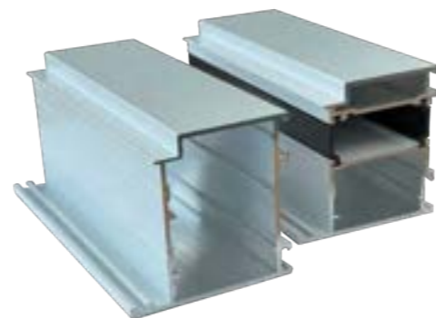
Verschil niet thermisch onderbroken kozijn (links) en thermisch onderbroken kozijn (rechts).
